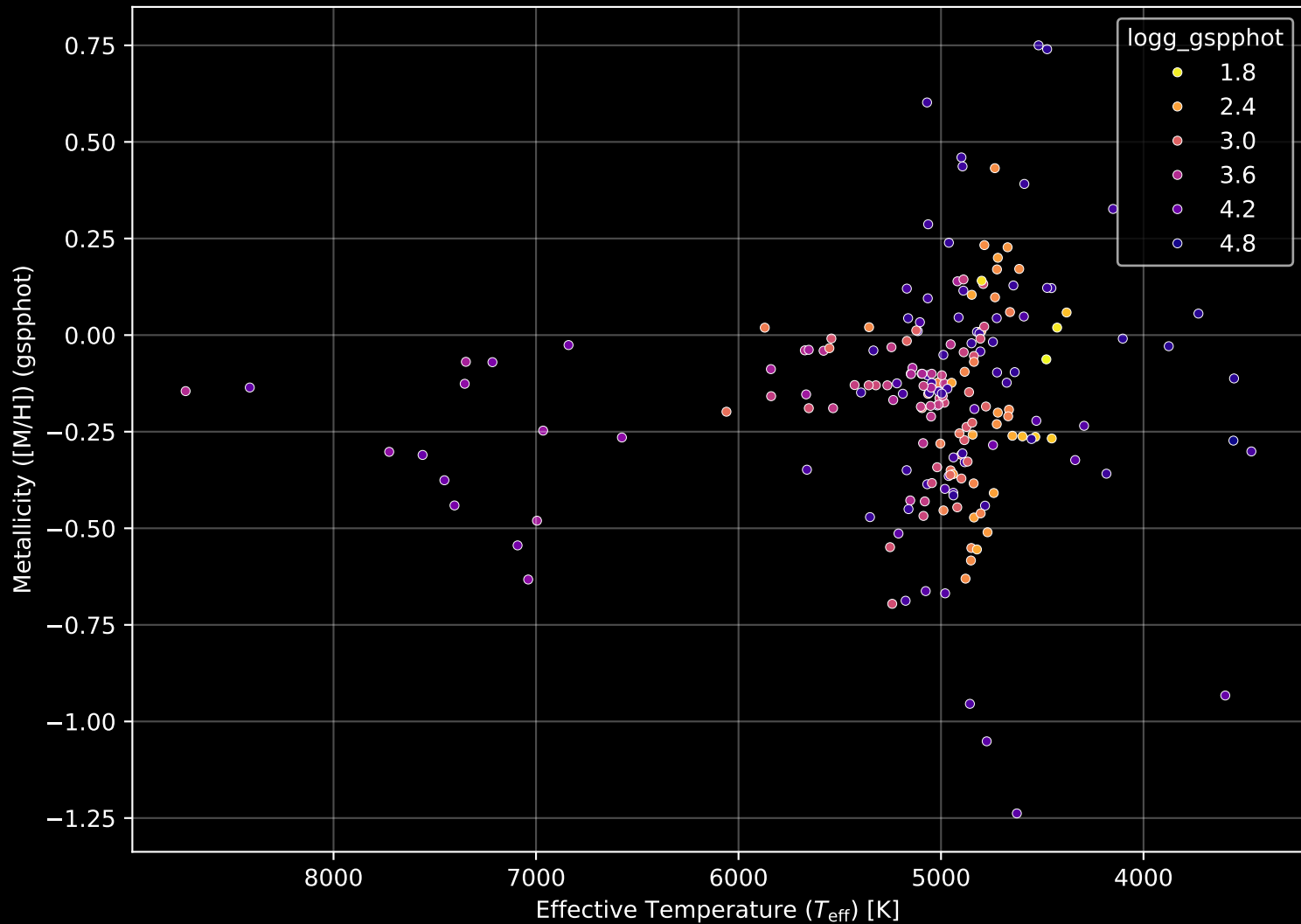
APOGEE DR17 Field: [K2_C16_204+27_btx] Stellar Population Parameters (n= 197)
